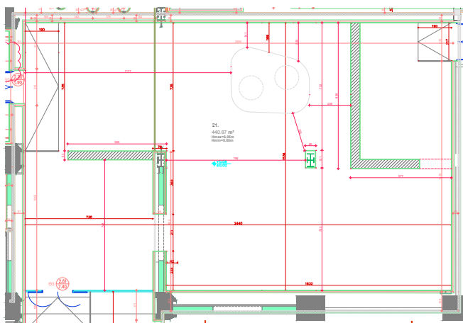
Κάτοψη Χώρου
