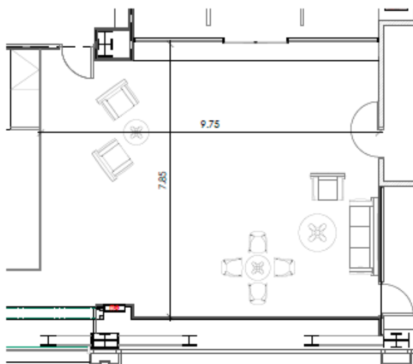
Κάτοψη Χώρου
