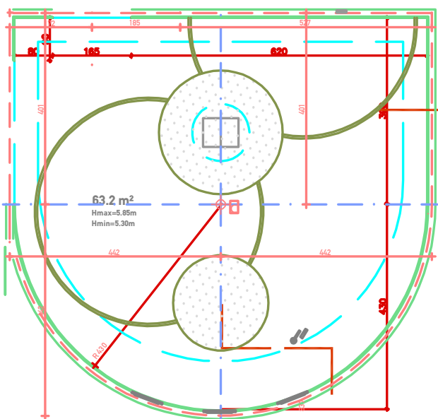
Κάτοψη Χώρου
