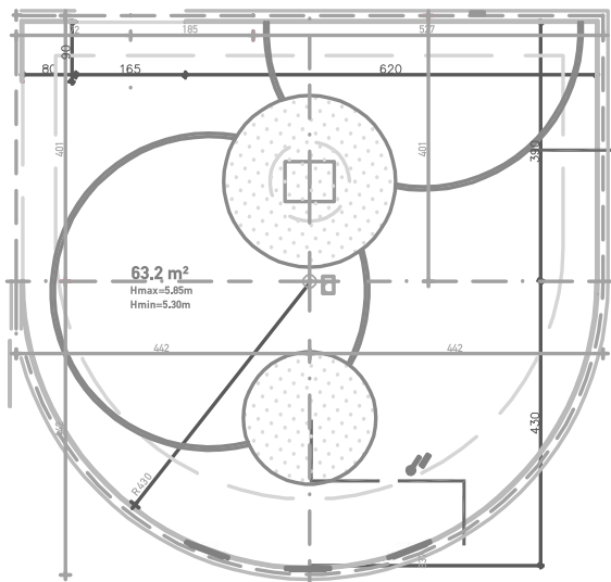
Κάτοψη Χώρου
