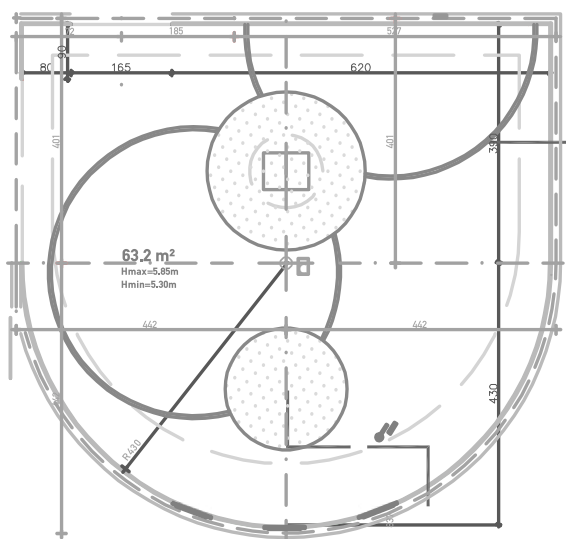
Κάτοψη Χώρου
